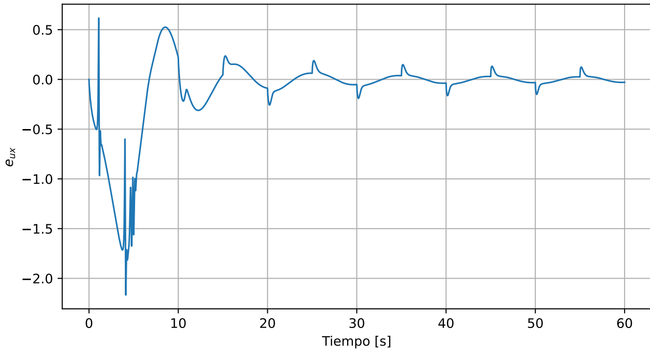
Error con tren de pulsos: u_x
